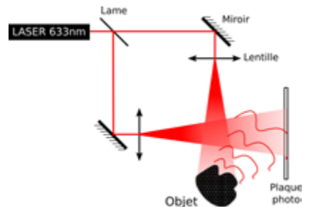
Figure 1. Montage dit « de Gabor » pour un hologramme observable en transmission.
