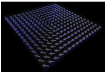
Simulation numérique d'un vortex magnétique.
