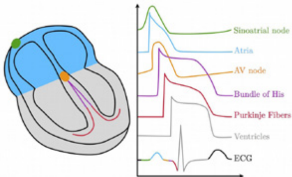
Potentiel électrique en divers endroits du cœur et électrocardiogramme (ECG)
