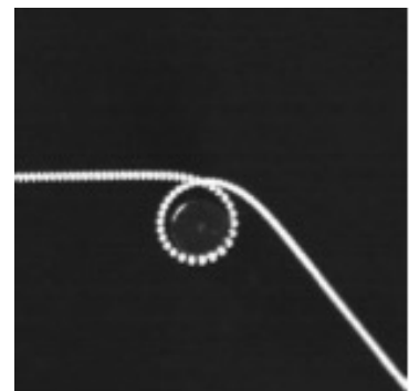
Fig. 1. Vue du dessus de la trajectoire d'une goutte d'oxygène liquide en caléfaction, en orbite autour d'un aimant (photo Keyvan Piroird).
