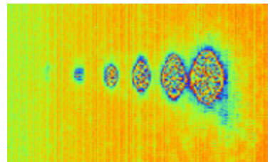
Dessin 3: Image moyenne de 6 sources de ^{14}\text{C} (ici en saturation pour l'étude du bruit).
