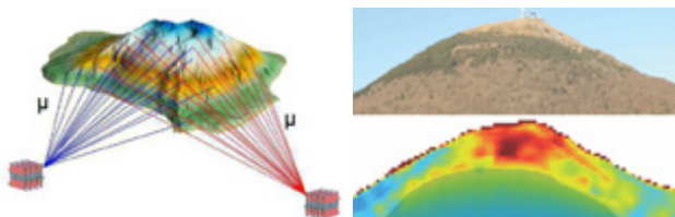
Dessin 4. Principe (gauche) et mesure (droite) de la densimétrie par muographie du Puy de Dôme, laissant apparaître la chambre magmatique.
